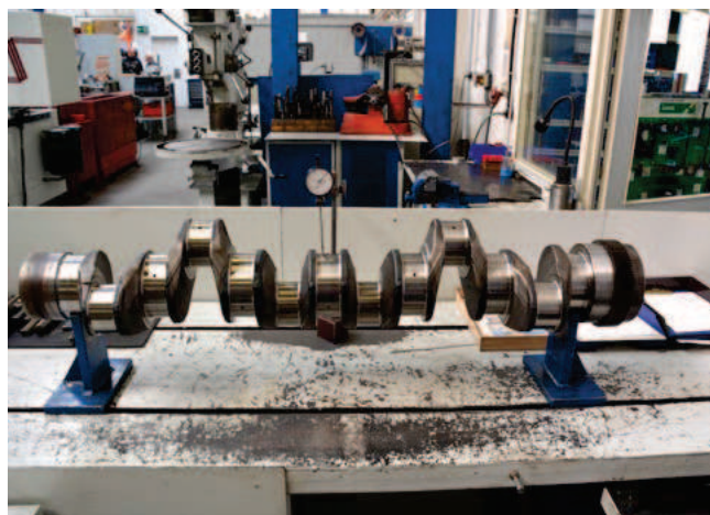
Zeitwertgerechte Reparatur, ob Kurbelwelle oder Zylinderköpfe, ist bei Motoren Eckenkamp tagtägliche Arbeit.
