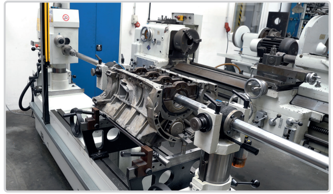
Oben: Hauptlagergassen-Bohrwerk
