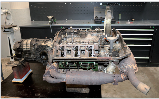
Oben: Ein Porsche 911er-Motor vor der Revision
